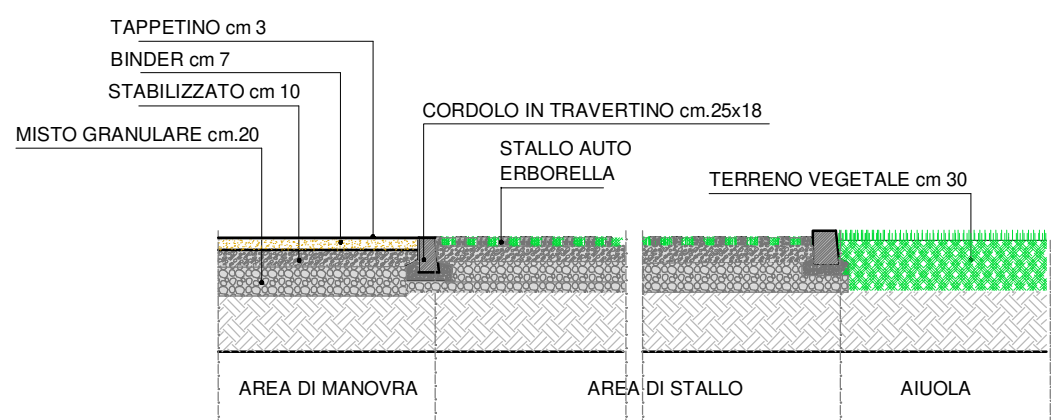
PARTICOLARE SEZIONE PARCHEGGIO SCALA 1:50
