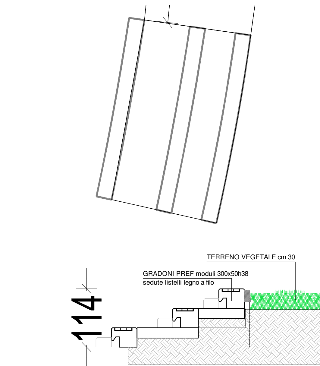
PARTICOLARE SEZIONE GRADONI CAVEA. SCALA 1
