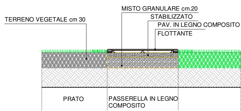
PARTICOLARE SEZIONE VERDE PUBBL. SCALA 1:50
