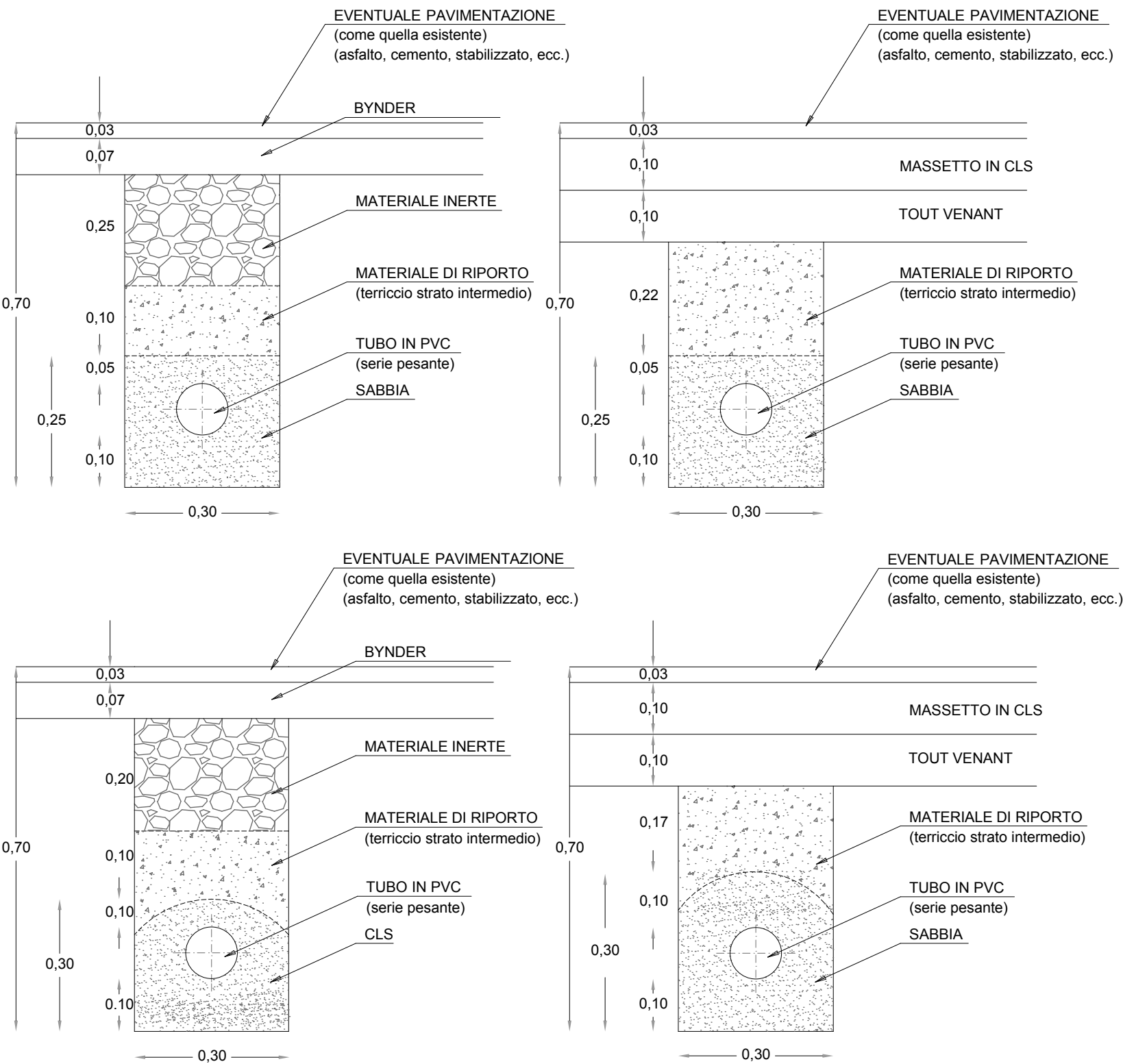
PRESCRIZIONI _SCALA 1:10
