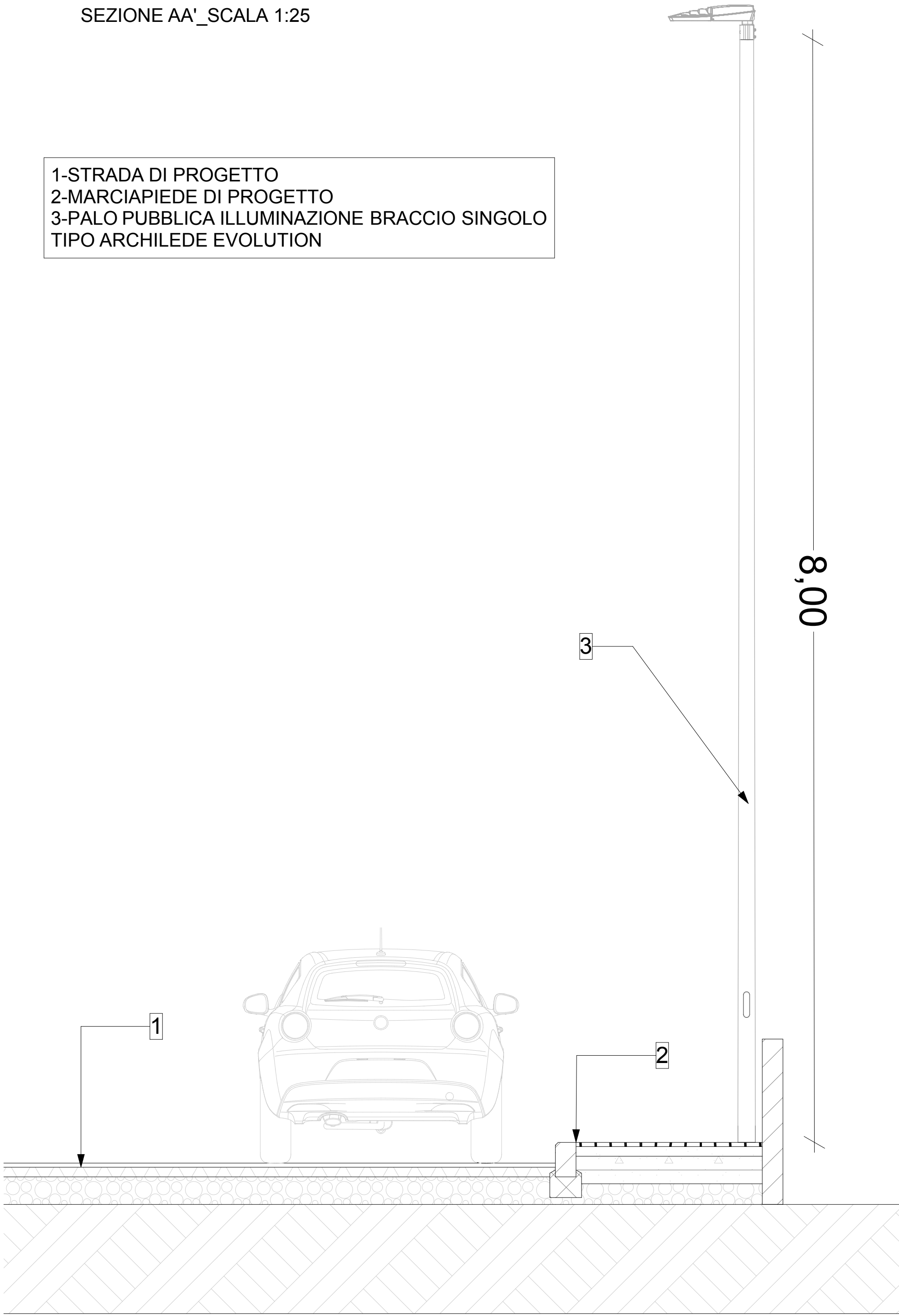
SEZIONE AA'_SCALA 1:25
