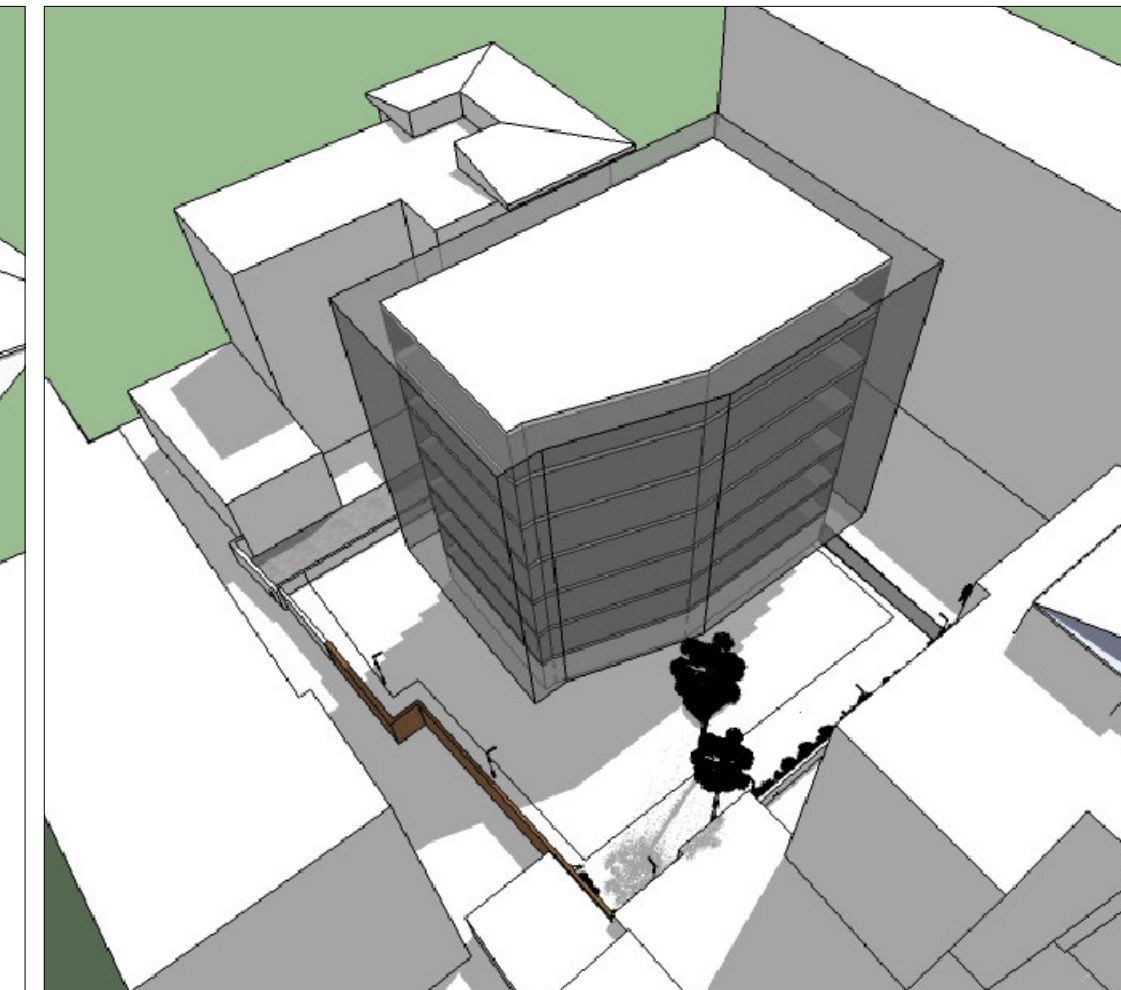
3) simulazione 3d vista aerea su lato interno edificio nuova costruzione
