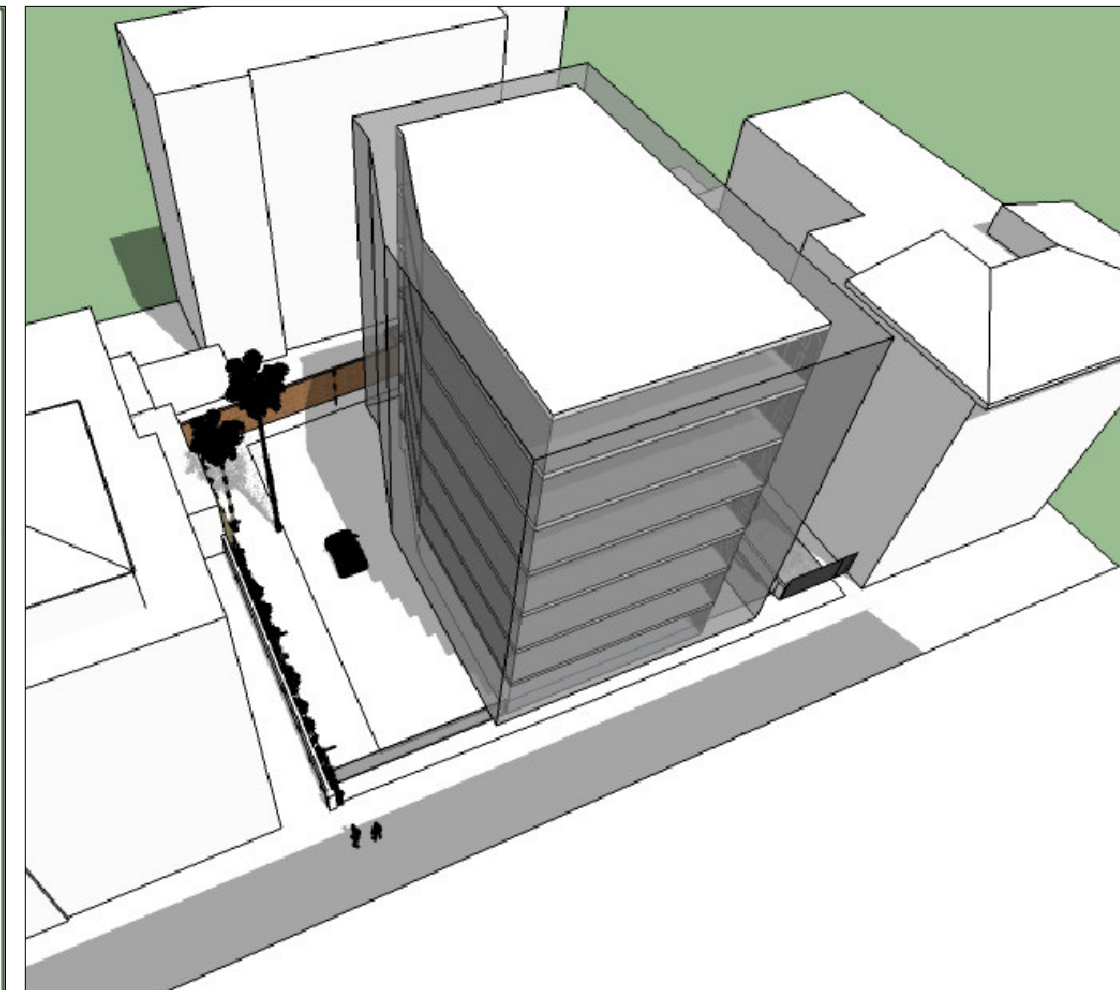
2) simulazione 3d vista aerea su via Piave edificio nuova costruzione
